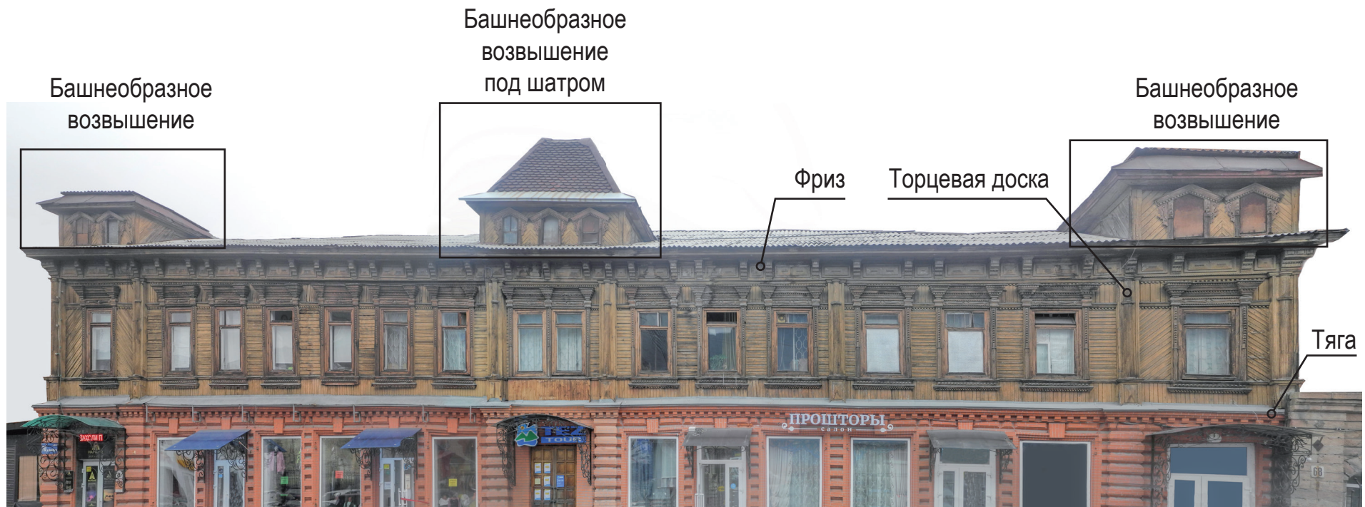
Южный фасад
